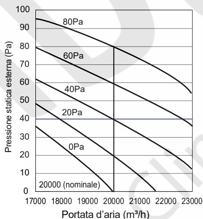
Curva delle caratteristiche della ventola 18HP
