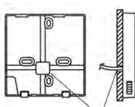
Foro nel muro e per i fili Diametro foro: Ø20mm
