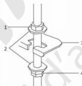
1 Dado 2 Rondella 3 Staffa di sospensione 4 Doppio dado
