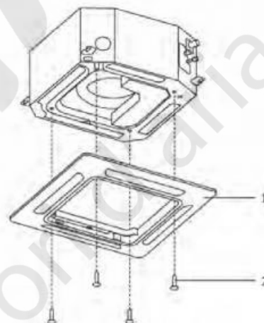
1 Pannello 2 Viti (M5) (fornite con il pannello)
