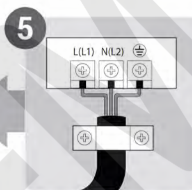
5 Collegare i cavi
