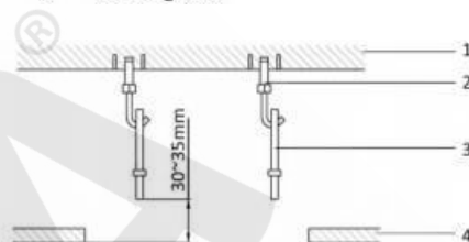
1 Lastra del soffitto 2 Gancio espandibile (opzionale) 3 Gancio per l'installazione (opzionale) 4 Cartongesso
