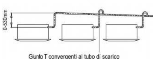
Giunto T convergenti al tubo di scarico
