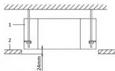
1 Unità interna 2 Cartongesso
