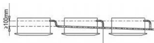
Giunto T convergenti al tubo di scarico
