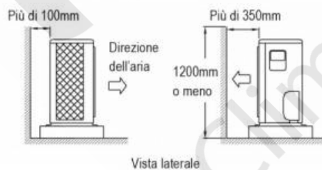
Vista laterale
