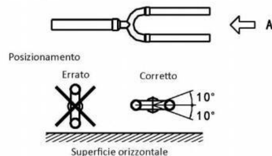
Giunto ad U
