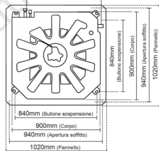
60K Modello Slim dimensione del foro del soffitto
