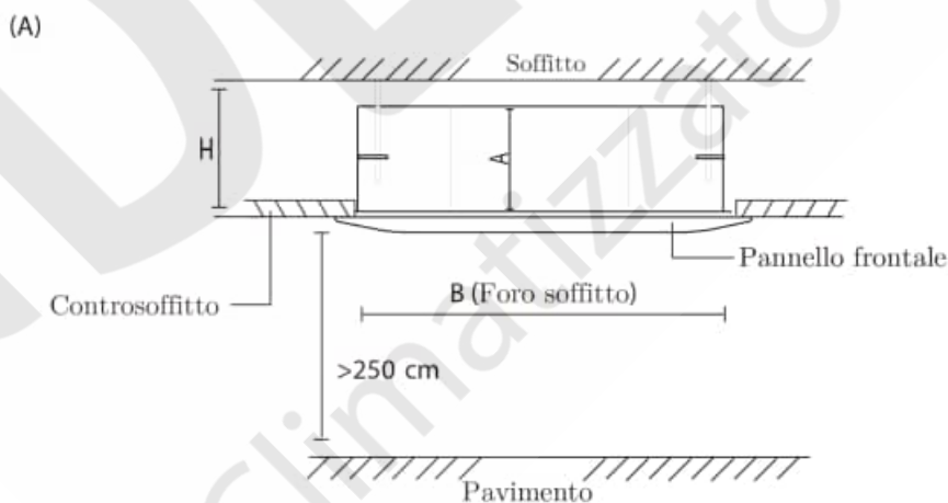
Distanza dal soffitto rispetto all'altezza dell'unità interna
