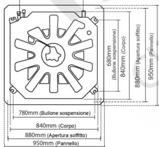
18K-48K Modello Slim dimensione del foro del soffitto
