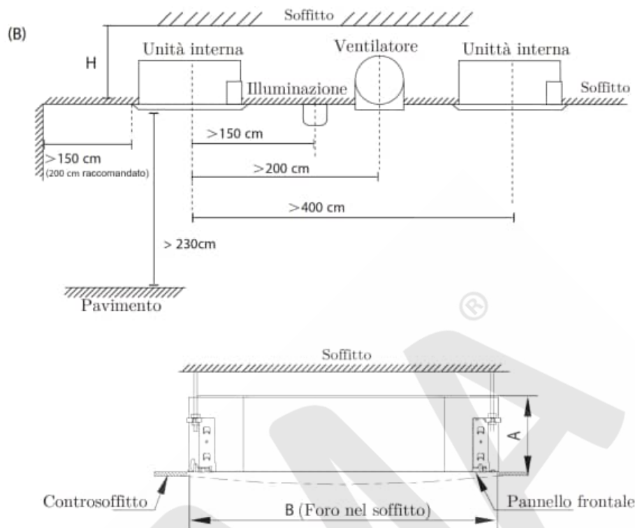
Distanza dal soffitto rispetto all'altezza dell'unità interna
