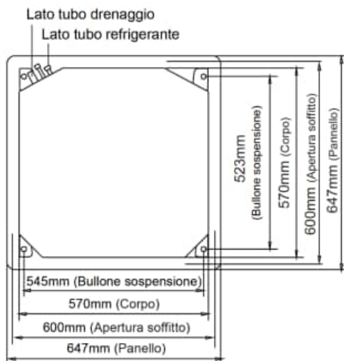
Modello Compatto dimensione del foro del soffitto
