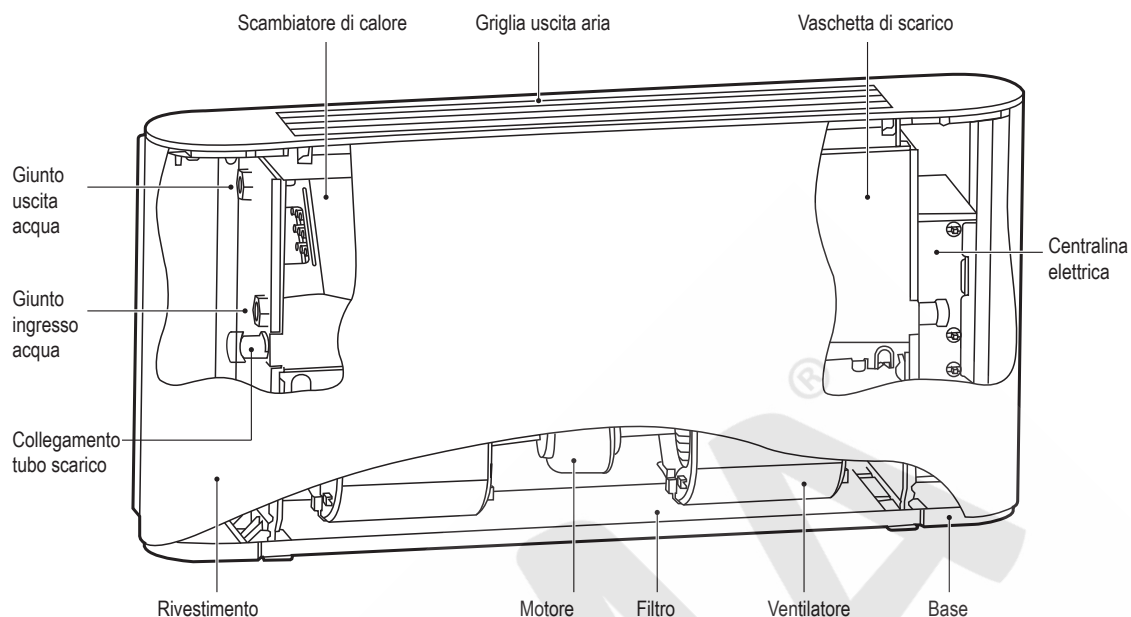
Figura 4-2 Schema dell'unità (esposta)
