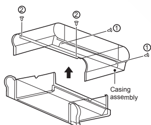
Figura 4-6 Rimozione del rivestimento
