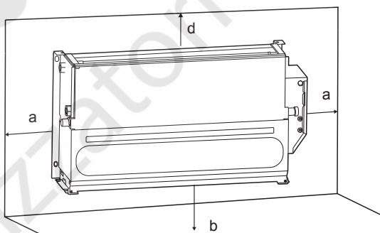
Figura 5-10 Montaggio di tipo verticale esposto
