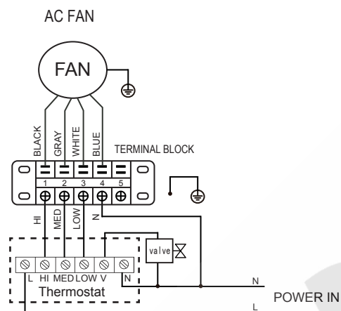
Figura 5-22 Schema dei cavi (VENTILATORE DA)
