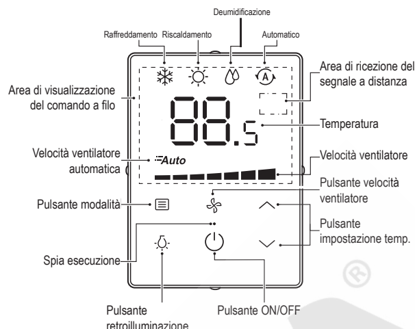
Figura 3-3 Pannello di controllo del comando a filo del fabbricante
