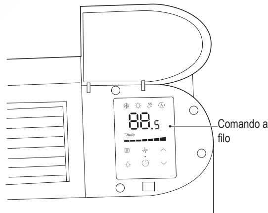
Figura 3-2 Dopo l'installazione del comando a filo
