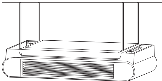
Figura 5-5 Schema del montaggio a soffitto esposto
