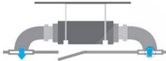
Presa d'aria posteriore e mandata diretta (STANDARD)
