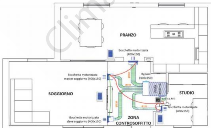
Presa d'aria tramite il controsoffitto
