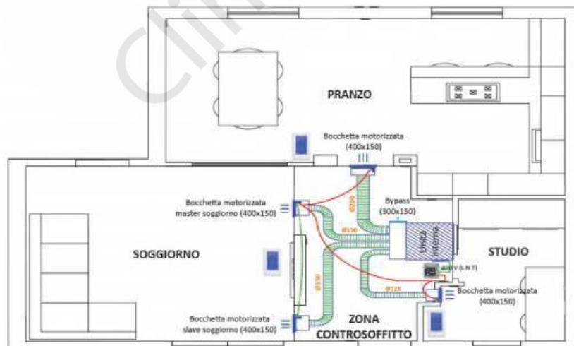
Presa d'aria tramite il controsoffitto
