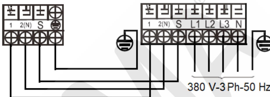
UNITA' ESTERNA
